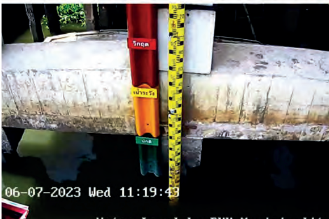
ระบบรายงานสถานการณ์ระดับน้ำ (ผ่านกล้องวงจรปิด)
