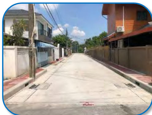
ปรับปรุงถนน คสล. บริเวณหมู่บ้านกฤษดานคร ซอยราชพฤกษ์ 29
